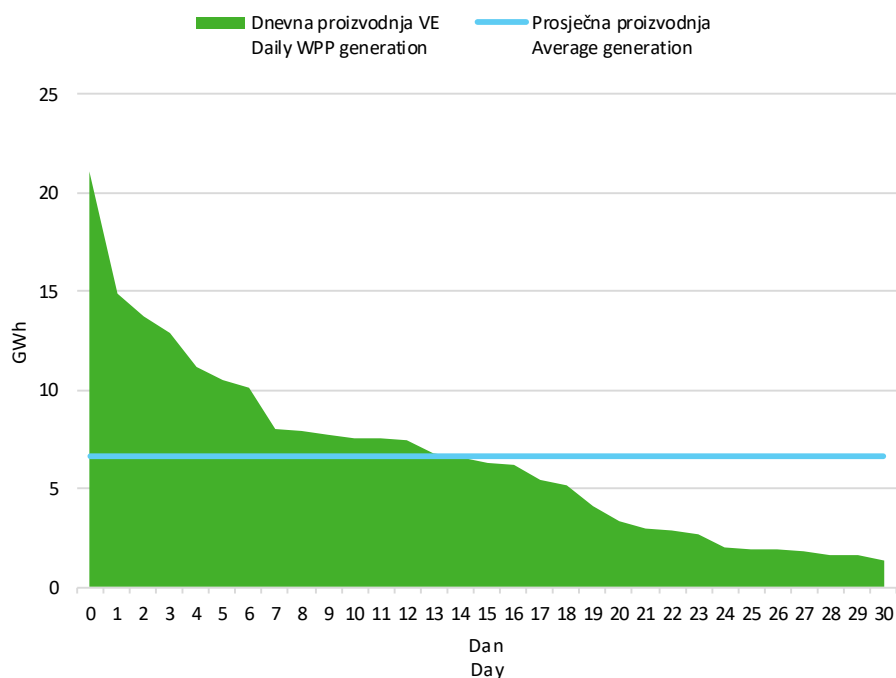
Slika 6 Krivulja trajanja dnevne proizvodnje vjetroelektrana u srpnju 2025. godine
