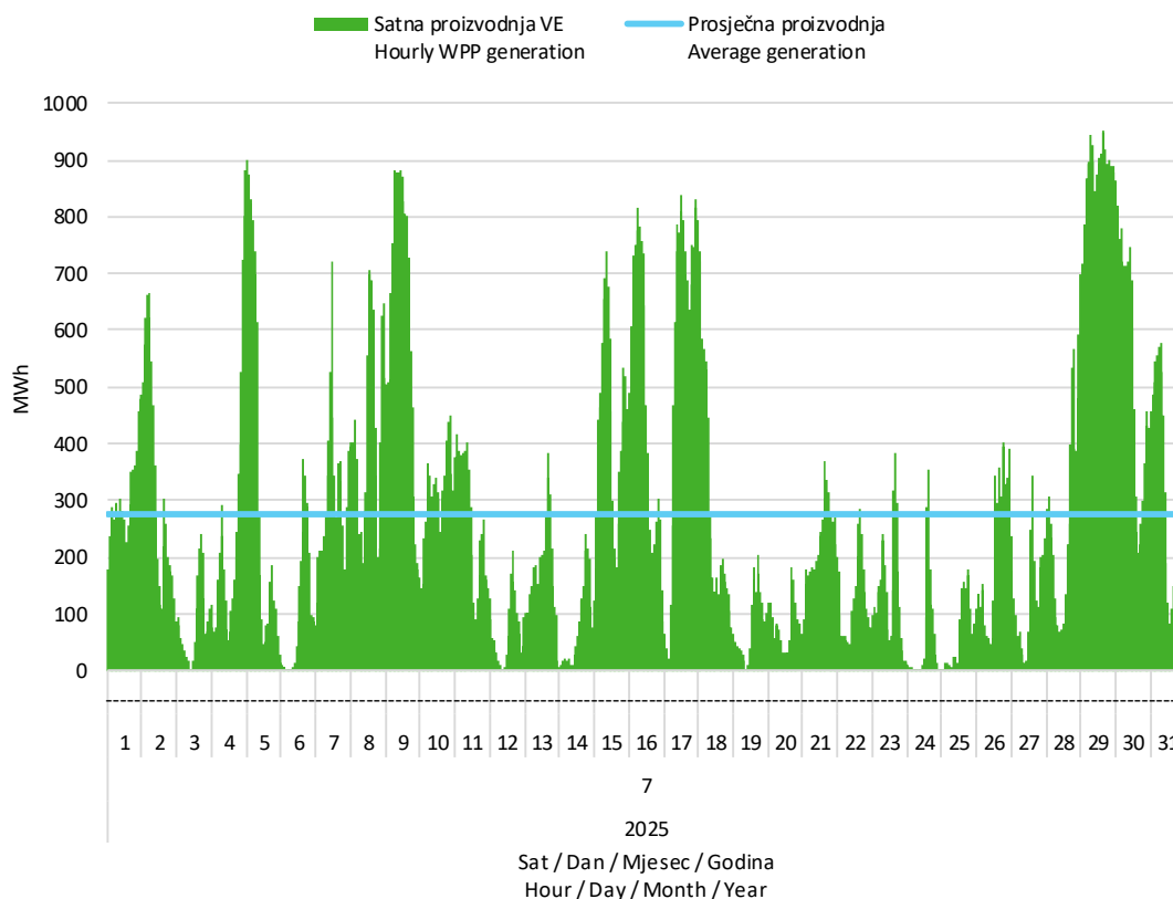
Slika 2 Satna proizvodnja svih vjetroelektrana u srpnju 2025. godine
