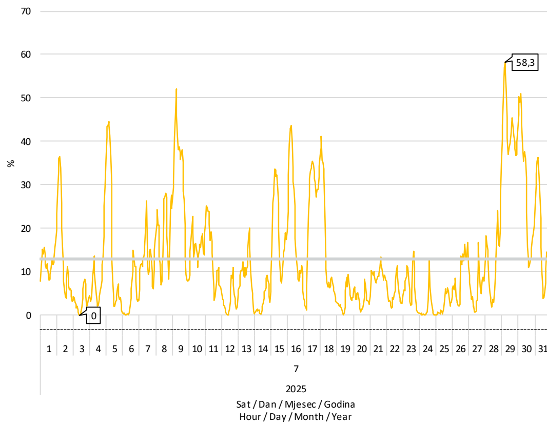
Slika 8 Udio proizvodnje vjetroelektrana u pokrivanju satnog opterećenja elektroenergetskog sustava u srpnju 2025. godine
