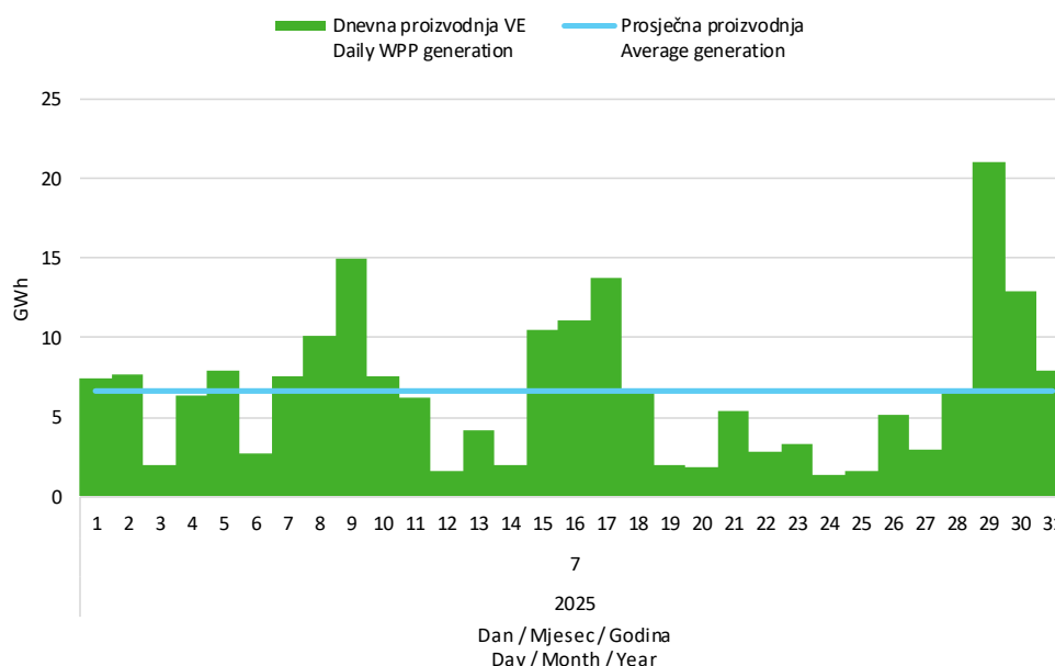
Slika 5 Dnevna proizvodnja svih vjetroelektrana u srpnju 2025. godine
