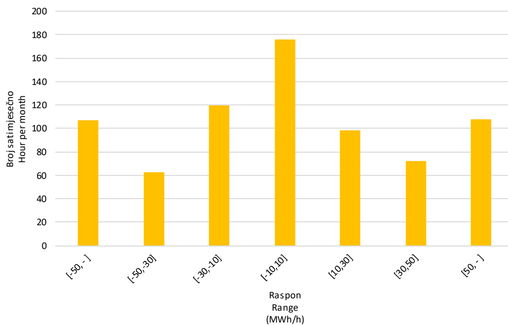
Slika 10 Statistička raspodjela satnih promjena proizvodnje VE u srpnju 2025. godine
