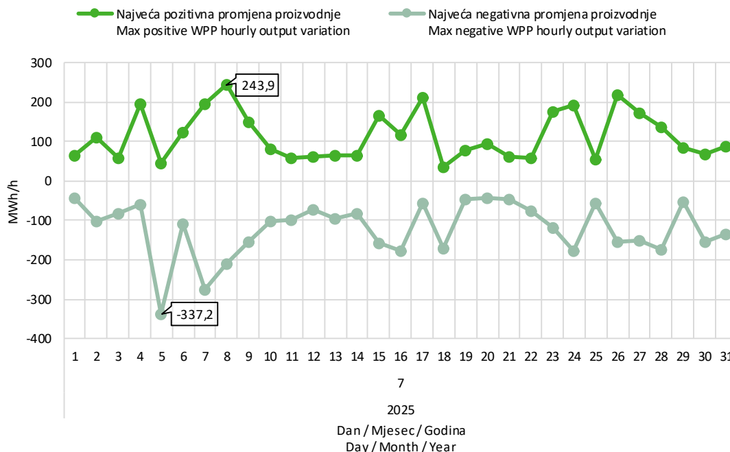
Slika 9 Maksimalna pozitivna i maksimalna negativna promjena satne proizvodnje VE u srpnju 2025. godine
