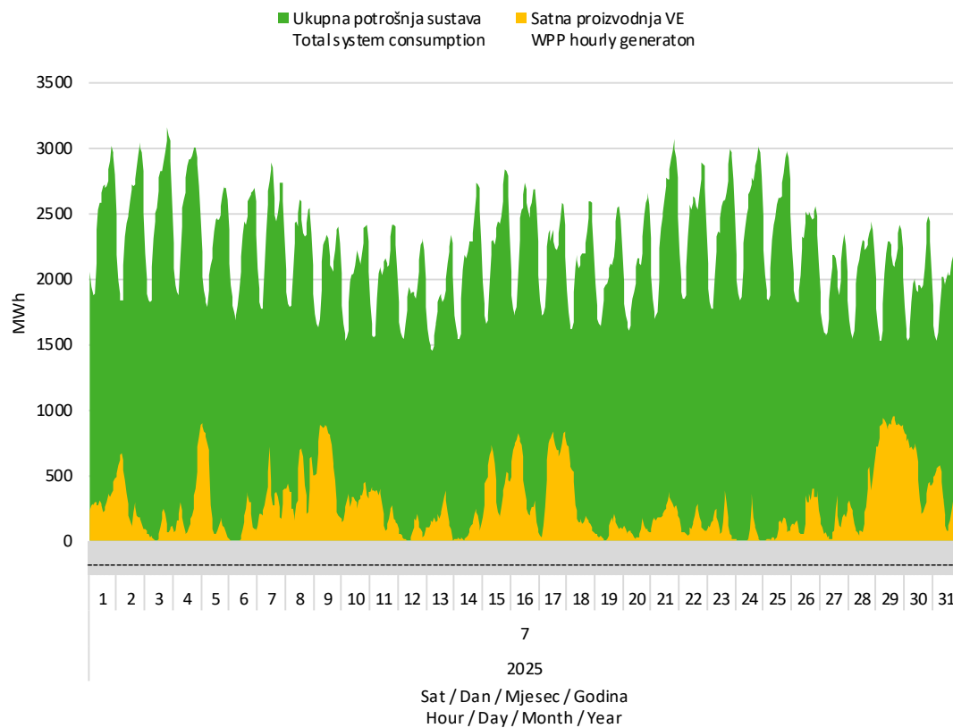
Slika 7 Usporedba satnog dijagrama opterećenja sustava i proizvodnje vjetroelektrana u srpnju 2025. godine
