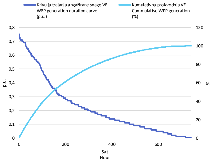
Slika 3 Krivulja trajanja angažirane snage svih VE i kumulativna proizvodnja VE u srpnju 2025. godine u jediničnim vrijednostima
